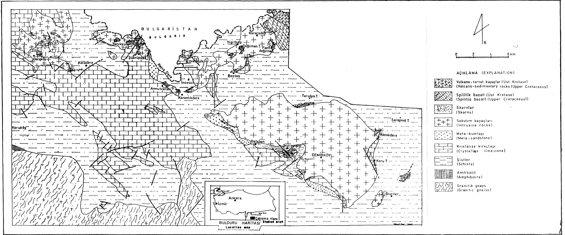
Şekil 1 : Istranca masifi jeoloji haritası (Ayhan ve diğerleri (1972) den değiştirilerek) Figure 1 : Geological map of the Istranca massif (Modified from Ayhan et al. (1972))
