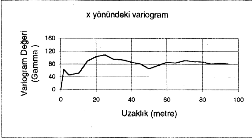
Şekil 4. Çevreleşmenin x,y,z yönlerindeki variogramlar ve uyarlanan model variogram.
