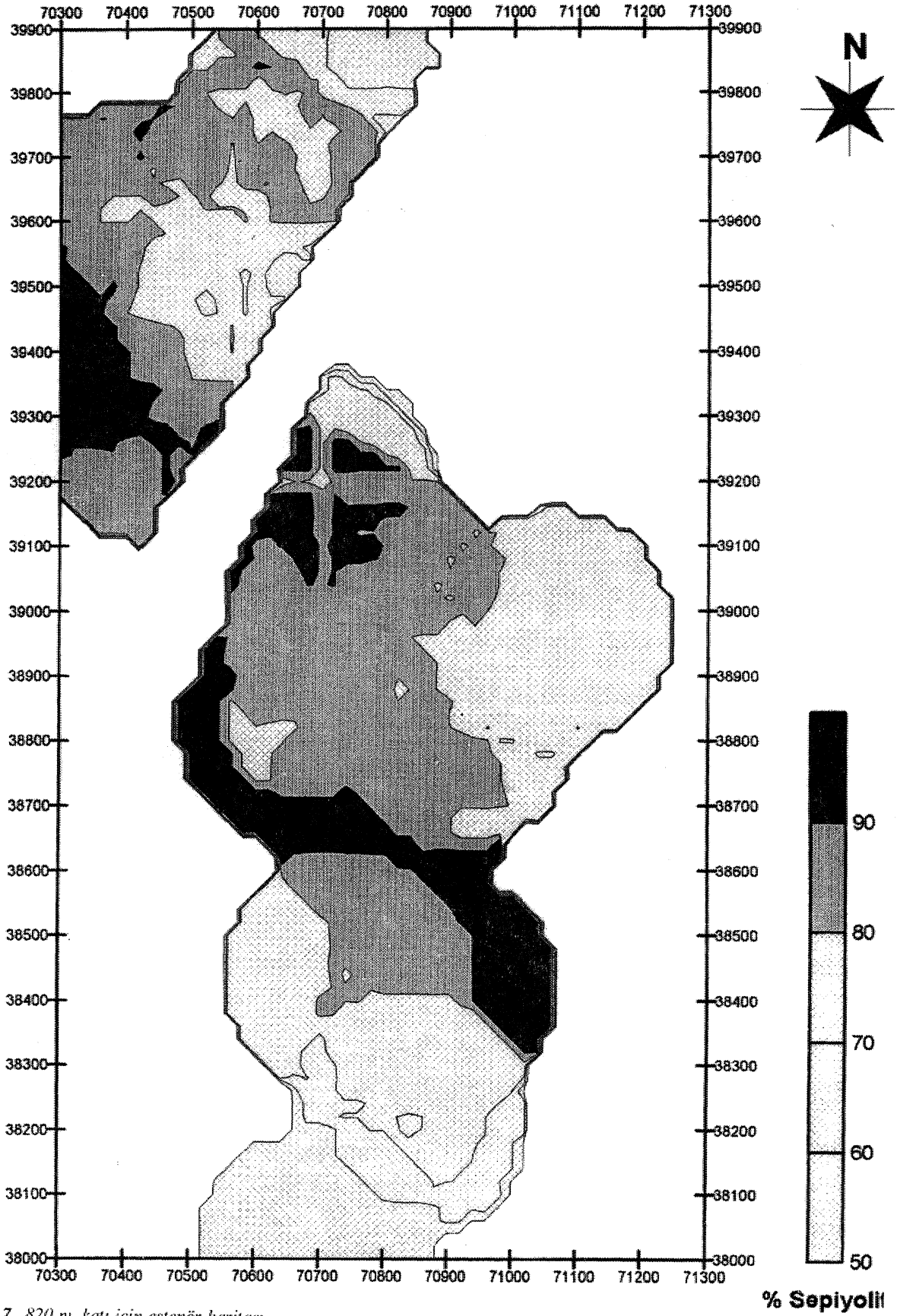
Şekil 7. 820 m. katı için eştenör haritası.
