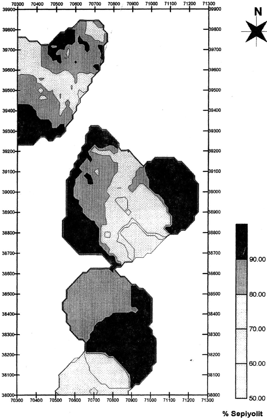
Şekil 8. 815 m. katı için eştenör haritası.
