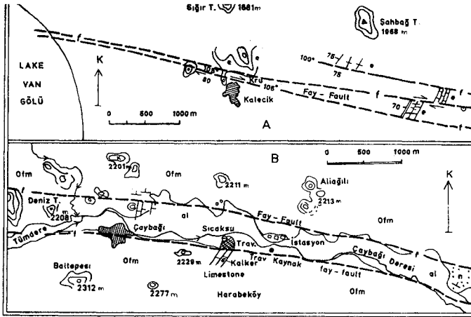
Sekil 5: III numaralı Fay zonunun batıda, Kalecik köyü yakınında (A) ve doğuda Çaybağı deresindeki (B) durumu. e-Eosen kalkerleri, Ofm-Ofiyolitik karmaşık, I-Fay, al-Allüvyon, n-Neojen, Trav-Traverten.
