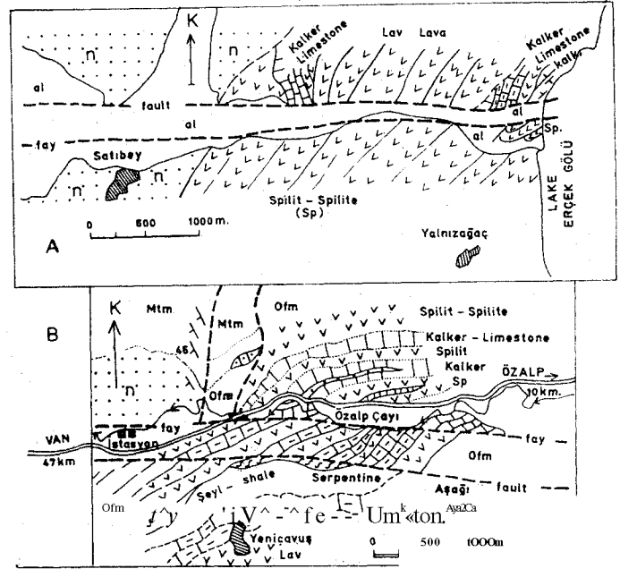
Şekil 3: II numaralı fay zonuna ait Erçek Gölü-Satibey köyü arası (A) ile Yeniçavuş köyü çevresinin (B) ayrıntılı jeolojik durumları, al-alüvyon, n-Neojen, Mtm-Metamorfik kayalar, Ofm-Ofiyolitik karmaşık, sp-Spilit.
