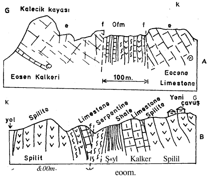
Şekil 4/A: III numaralı fay zonunun Kalecik köyünde, Kalecik kayası kuzey kenarındaki görünümü; 4/B: II numaralı fay zonunun Yeniçavuş köyü yakınındaki görünümü. f-Fay düzlemi, e-Eosen, Ofm-Ofiyolitik karmaşık.
