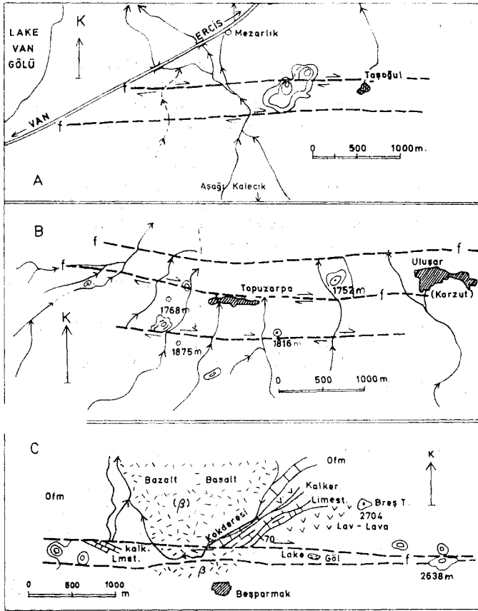
Şekil 2: I numaralı zona ait fay parsalarına doğrultu atımlı-sağ yönlü olduklarını belirleyen dere yataklarının (A, B) ve tabaka serilerinin (C) ötelenmeleri. Ofm-Ofiyolitik karmaşık, Kalk-Kireçtaşı.
