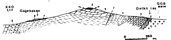
Şekil 10: Gögebakan mevki-Deliklitaş arasında jeolojik kesit. 1 — Granodiyorit, 2 — Granat fels, 3 — Alt mermer, 4 — Şistler, 5 — Bolkardağ mermerleri, 6 — Alihoca ofiyolit serisi, 7 — Üst Maestrihtien taban konglomerası, 8 — Alt Eosen taban konglomerası.
