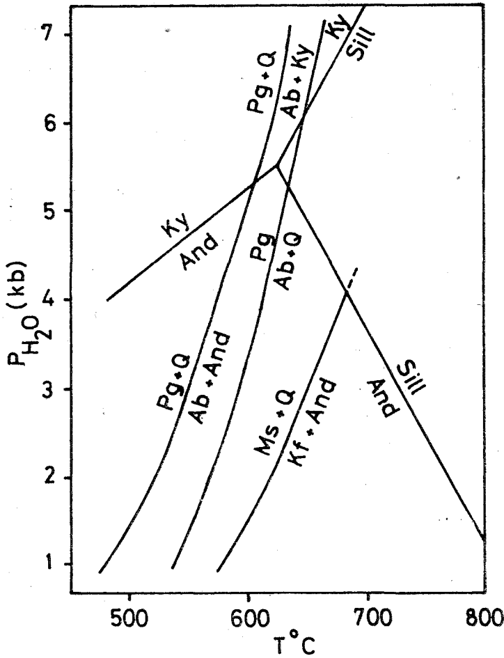
Sekil 3: Paragonit -f- kuvars ve paragonit duraylılıklarının üst limitindeki P_{H_2O} - T^{\circ}C ilişkileri (Chatterjee, 1970) ile muskovit -f- kuvars (Althaus ve diğerleri, 1970) ve çeşitli Al_2SiO_5 polimorfizmlarının duraylılıklarının (Richardson ve Gilbert 1969) kıyaslanması.
