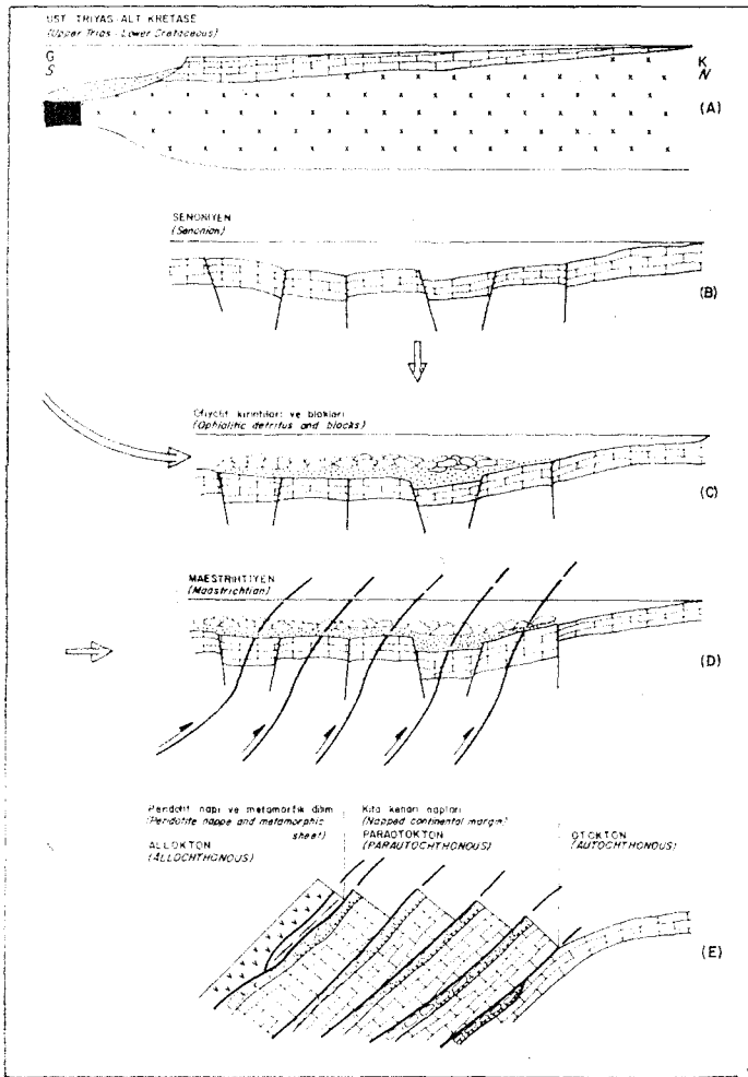
Şekil 2: 'Üst Triyas-Maestrihtiyen zaman aralısında Aladağlar'ın yapısal evrimi.
