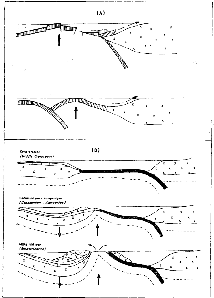
Şekil 3: Üst mantonun ve okyanus kabusunun diyapirik yükselmeye bağlı olarak gerçekleşen ofiyolit yerleşmesi modelleri (A: Gass et. ali., 1975; B: Stonoiey, 1975).
