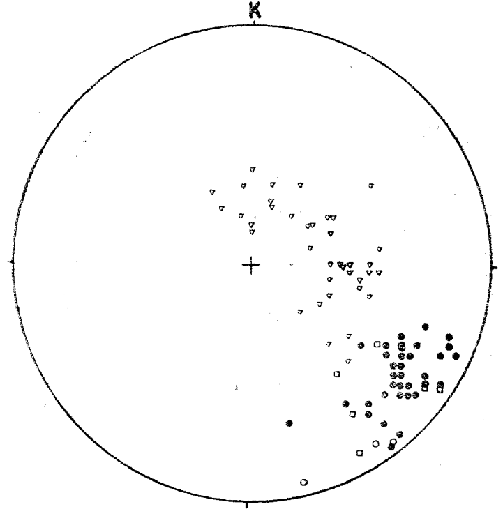
8: Mermerlerde tabakalanma düzlemlerinin (üçgenler) ve çizgisellik yönlerinin (küçük daireler) kutupları, içi boş kareler glaukofan-lavsonit zonu metacörtlerindeki çizgisellik, içi boş daireler ise Göynücek güneyindeki büyük mermer yüzleğindeki çizgisellik kutuplarını belirtir (Schmidt ağı)
