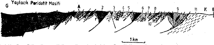
Şekil 5: Gümüşyeniköy yöresindeki ofiyolitli melanjın iç yapışım acıklıyan somatik kesit: V25.000 ölçekli jeoloji haritasından alınmıştır; (1) amfibolit; (2) ultramafik kaya; (3) şeyl; (4) radyolarial çört; (5) yabancı kireçtaşı merceği; (6) bazik volkanik kaya; (7) grovak; (8) pelajik kireçtaşı; (9) yeşilgist; (10) manganez - çört kayası; (11) lavsonit zona şistleri.
