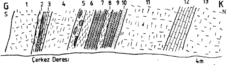
Şekil 4: Başlangıç metamorfizması gösteren ofiyolitli melanja öze volkanotortullarda tipik bir yerel kesit (Ketenlik köyünün 2 km kuzeyindeki Çerkez deresinde ölçülmüştür). (1) Yapısız, yeşil spilit; (2) yeşil şeyi; (3) pembe, ince tabakalı kireçtaşı; (4) ezilmiş (sheared) yeşil şey ve acık yes» spilit (K731/3), feldieparca çengin traktik bazalt, az miktarda bulunan ojitler sodik piroksen tarafından ornatılmış; (5) kireçtaşı Tp çört parçacıklarının volkanik, yeşil bir hamurda yer aldığı konglomera; (6) mavi-eri şeyi; (7) tabakalı, kırmızı radyolaryalı çört; (8) mavi-yeşil ve kırmızı şeyi; (9) tabakalı, kırmızı radyolaryalı çört; (10) iri taneli grovak (K731/1): iri (>1mm), köşeli kuvars, plajiyoklaz, kalsit, şey ve az oranda epidot, garnet ve klorit parçacıklarından yapılmış olup klastik kuvars parçacıkları ince taneli agregatlar biçiminde yeniden kristallenmiş; (11) yeşil spilit; (12) ince tabakalı kireçtaşı; (13) yapısız yeşil spilit (K/730): ojitler, yeşil renkli sodik piroksen damarlarıyla kesilmiş» ayrıca bol miktarda aragonit ve kuvars damarları var.
