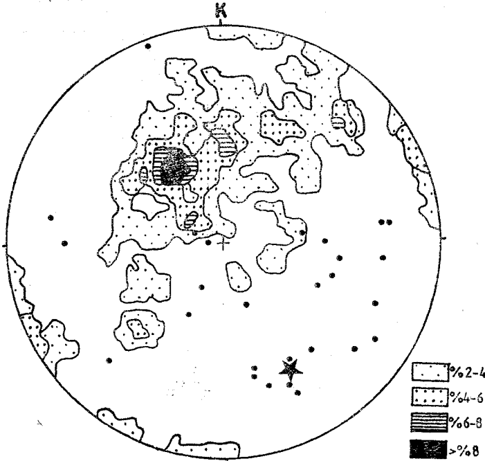
7: Bevez bölgesi glaukofan-lavsonit zonu mavişistlerinde küçük kıvrım eksenleri (küçük daireler) ve yapraklanma, düşlemleri kontur diyagramı (176 ölçü, konturlar yüzde 2, 4, 6 ve 8 yoğunluklarında çizilmiştir, Schmidt ağı). Yıldız ana kıvrım ekseninin kutbunu gösterir.
