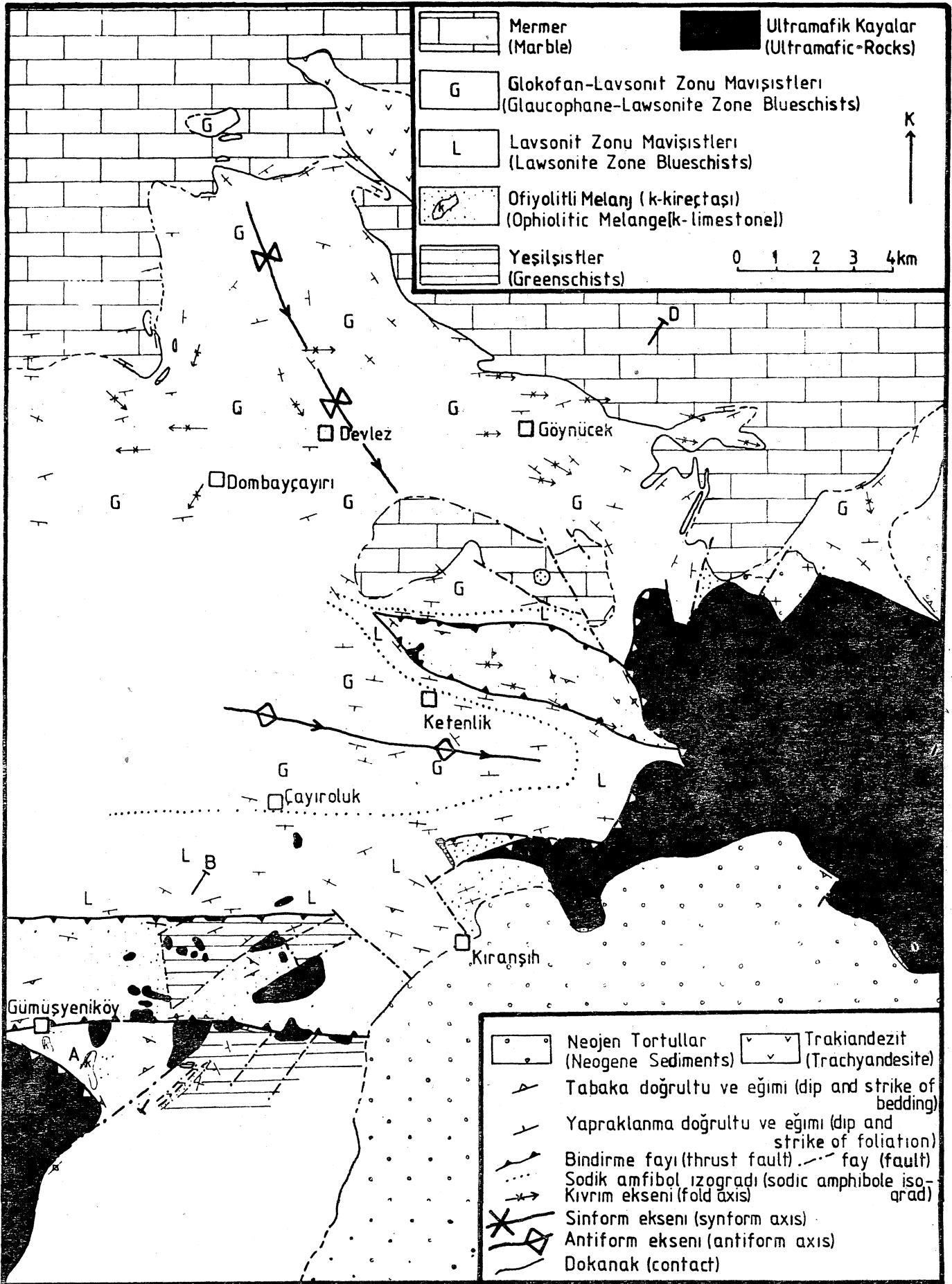
Sekil 2: Tavşanlı kuzeydoğu bölgesinin jeoloji haritası. Figure 2: The geological map of Northeast Tavşanlı region.
