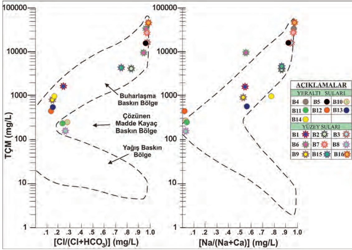
Şekil 7. Yüze ve yeraltı sularının Gibbs diyagramında gösterimi.
