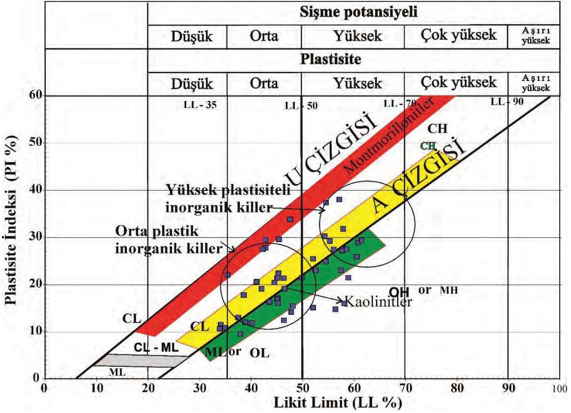
Şekil 9. Güdül zemin örneklerinin plastisite indisi-likit limit değerlerine bağlı şişme potansiyeli grafiğinde dağılımı (Daksanamurty ve Raman 1973' ten değiştirilerek alınmıştır).
