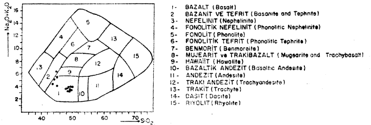
Şekil 11: Volkanitlerin alkali-silis içeriğine göre adlandırılmaları (Cox ve diğerleri 1979).
