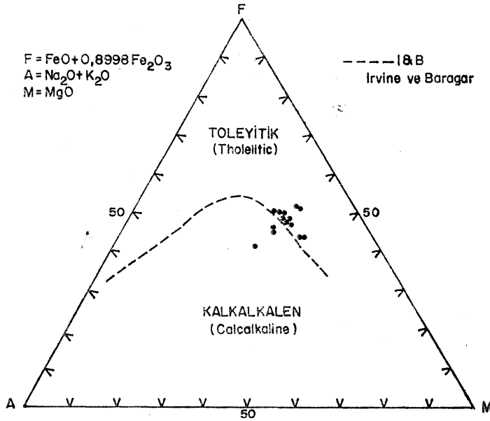
Şekil 6: YoUmmnitrerin AFM diyagramı
