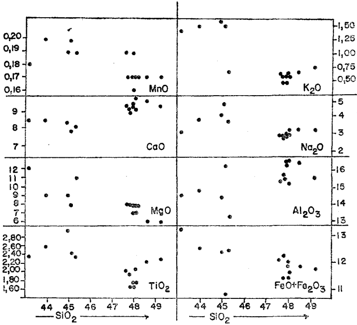
Şekil 12: Volkanitlerde oksitlerin SiO_2 değerlerine göre değişimi
