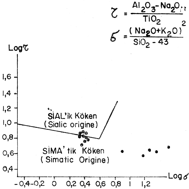
Şekil 9: Volkaniklerde \log T nun \log S ya göre değişimi Gottini, 1868, 1969)
