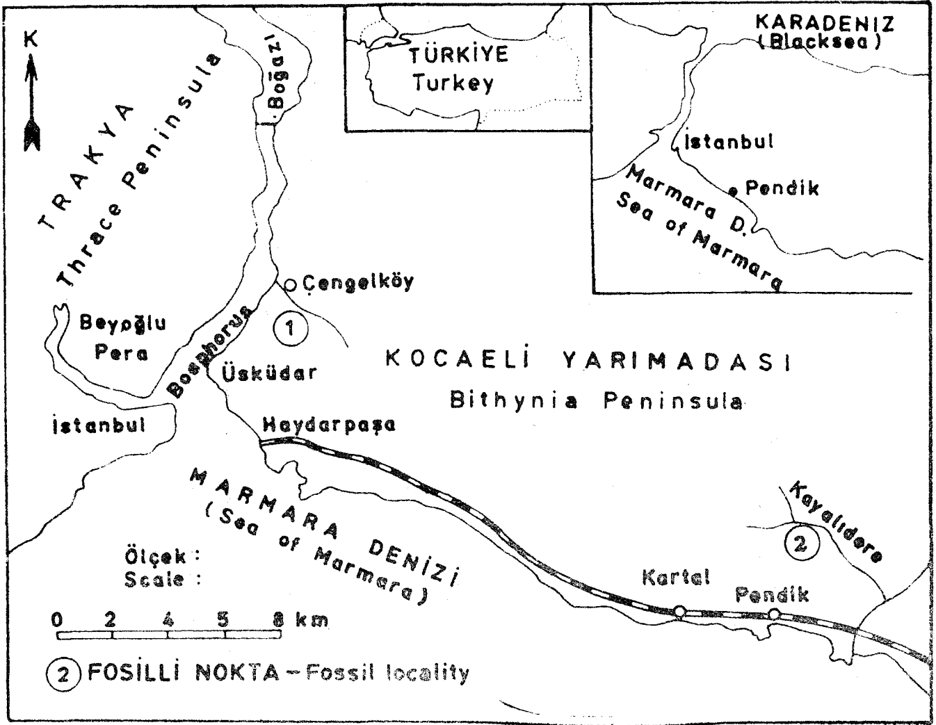
Şekil 1: İstanbul boğazı ve çevresinde Ordevisiyen-Silüriyen sınırı fosilli noktaları, daire içinde 1 ve 2,
