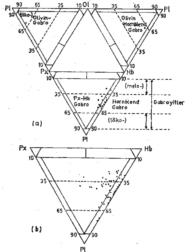
Şekil 2 : Kayaçların piroksen, plajiyoklaz, hornblend ve olivin içeriklerine dayanan IUGS sınıflandırması.
