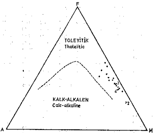
Şekil 4 : Örneklerin AFM diyagramında dağılımı (Irvine ve Baragar, 1971).
