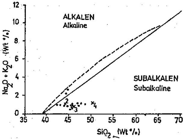
Şekil 3 : Gabro örneklerinin alkali-siyis içeriğine göre sınıflandırılması.
