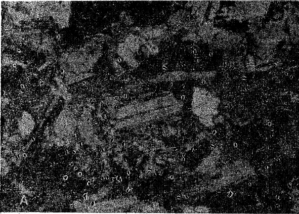
Şekil A : Homblend-gabro mikrofotografında plajiyoklaz kristalleri aîbit, karlsbad ikizlenme göstermekte, idiomorf ve hipidiyomorf plajiyoklazlarda yönlenme görülmektedir, Homblendler plajiyoklaz kristalleriyle intergranular dokudadır. Örnek no: 187, SW of Çamsan, Ânaizör ile, x35.
