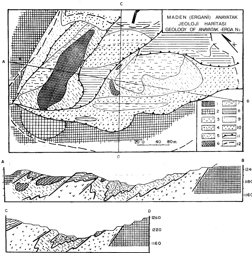
Şekil 4: Maden (Ergani) Anayatak Jeoloji haritası; 1 - Serpantinit, 2 - Gabro, 3 - Diyabaz, 4 - Cevherli diyabaz, 5 - Piritli fiörtler, 6 - Manyetitli klorititler, 7 - Cevherli siyah samurtaşları, 8 - Kırmızı-yeşil «amurtaşları, 9 - Bozunmuş serpantinit, 10 - Demir şapka, 11 - Bindirme, 12 - Asık işletme sınırı.
