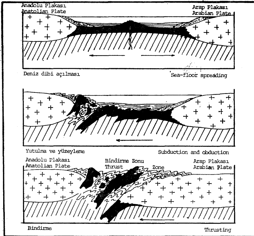
Şekil 9: Güneydoğu Anadolu bindirme kuşağının oluşum ve ofiyolitlerin üst bindirme ile yüzeylenmesinin şematik açıklanması.
