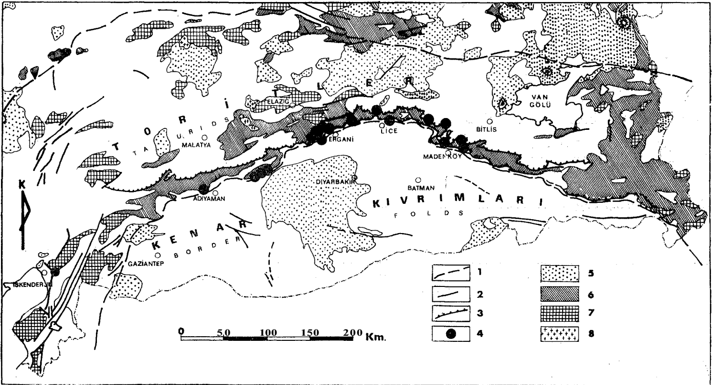
Şekil 1: Güneydoğu Anadolu'daki tektonik birimler ve bakır yataklarının dağılımı. Harita, Ketin 01966'den sadeleştirilerek alınmış, üzerine bölgenin bakır yatakları işlenmiştir. 1 — Tektonik birliklerin sınırları, 2 — Normal ve ters faylar, 3 — Bindirmeler, 4 — Bakır yatakları, 5 — Tersiyer ve Kuvaterner volkanik kayalar, 6 — Radyolarit fasiyesi (renkli melanj), 7 — Alpin bazik intrüziyel kayalar, 8 — Alpin granitik kayalar.
