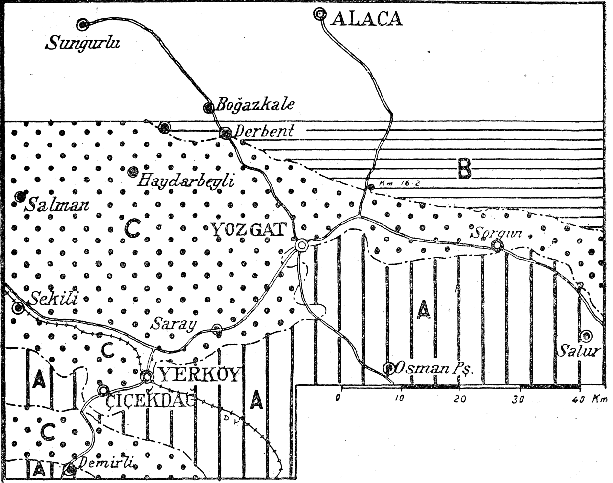
Şek. 2. Yozgat bölgesinin jeolojik anahatları. (A: Metamorfik - kristalin masifler, B: Serpantin ve radiolaritli Üstkretase, C: Tersier ve volkanik teşekkülât).
