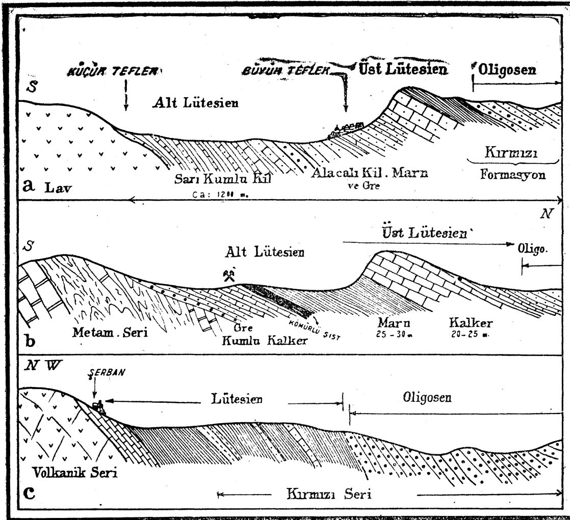
Şek. 4. Yerköy - Çiçekdağ bölgesinde lütésien tabakalarının detaylı kesitleri, a: Teflek kesiti, b: Arabm köyü kömür madeni kesiti, c: Şerban kesiti.
