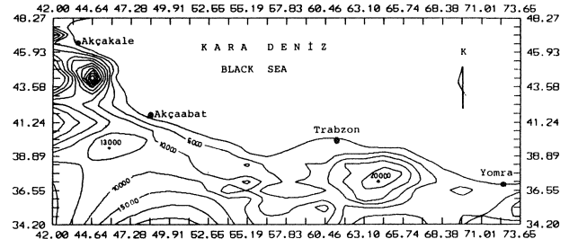
Şekil 4. Mn-dağılım haritası (Konturlar 500 ppm 1 de bir geçirilmiştir) yatay ve düşey rakamlar koordinat değerlerini göstermektedir.
