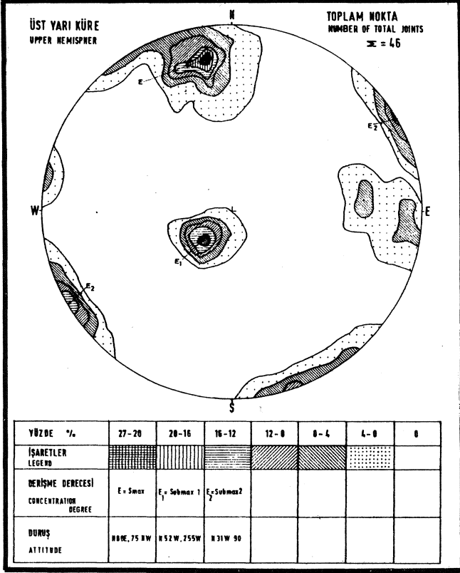
Şekil 4: Görmel formasyonundan ölçülmüş eklemlerin eşit alan izdüşümü.
